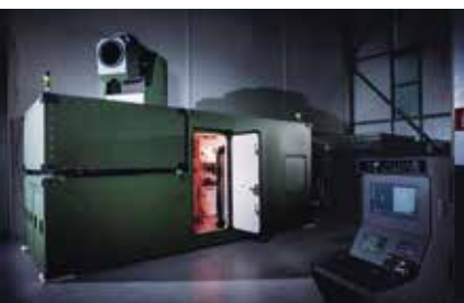
Rechts: Mit dem kleinen Laser Milos zerstört ein Bundeswehrtechniker in Meppen eine Mine
